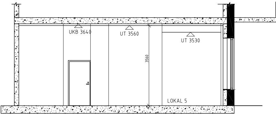
SEKTION E-E
