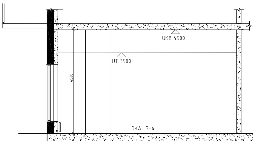
SEKTION G-G
