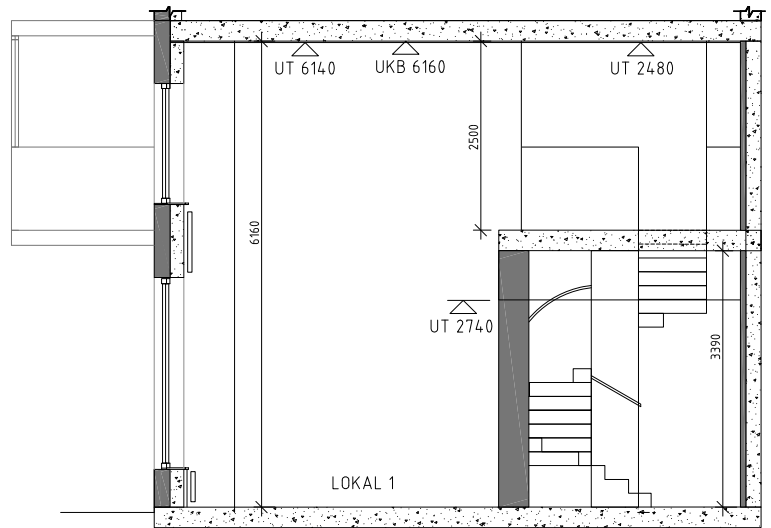
SEKTION A-A
