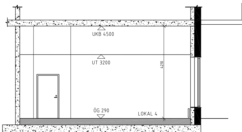
SEKTION D-D
